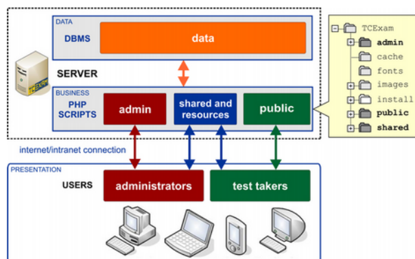
Figura 1: Struttura di TCEExam
